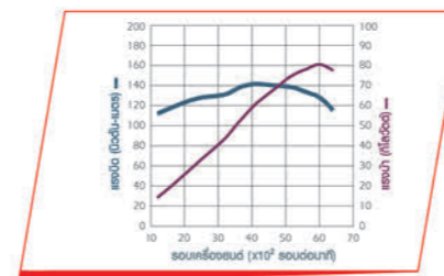
เครื่องยนต์ 1.5L 4 สูบ 16 วาล์ว DOCH ทำถึงกำลังสูงสุด 80 กิโลวัตต์ (109 แรงม้า) ที่ 6,000 รอบต่อนาที แรงบิดสูงสุด 141 นิวตัน-เมตร (14.4 กก.-ม.) ที่ 4,200 รอบต่อนาที
